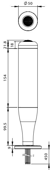
A-MOUNT
